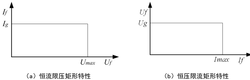
恒流限压与恒压限流矩形输出特性
